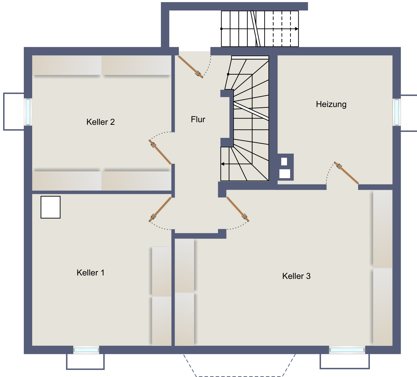
Kellergeschoss
